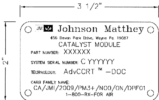
DOC Module
